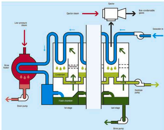
Fig. 3. MSF simple scheme (Palenzuela, Alarcón-Padilla, & Zaragoza, 2015).
