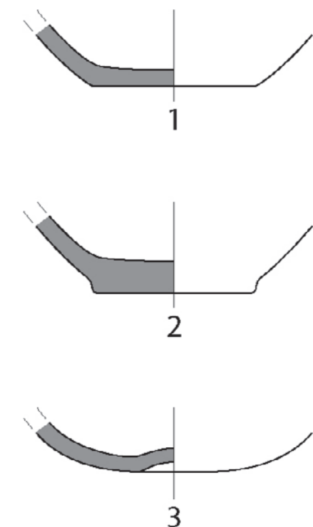
Slika 2.4. Tipovi dna: 1 ravno jednostavno, 2 ravno naglašeno, 3 pupčasto.
