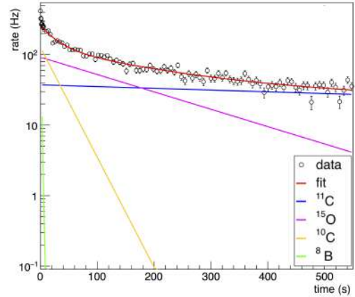
(d) ZEBA phantom: 10^9 incident protons
