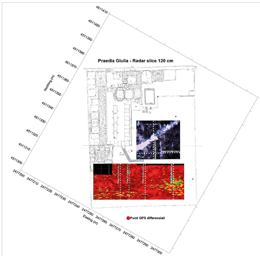
fig. 5. Mappa Praedia Iuliae Felicis: GPR-Slices Z=120 cm.
