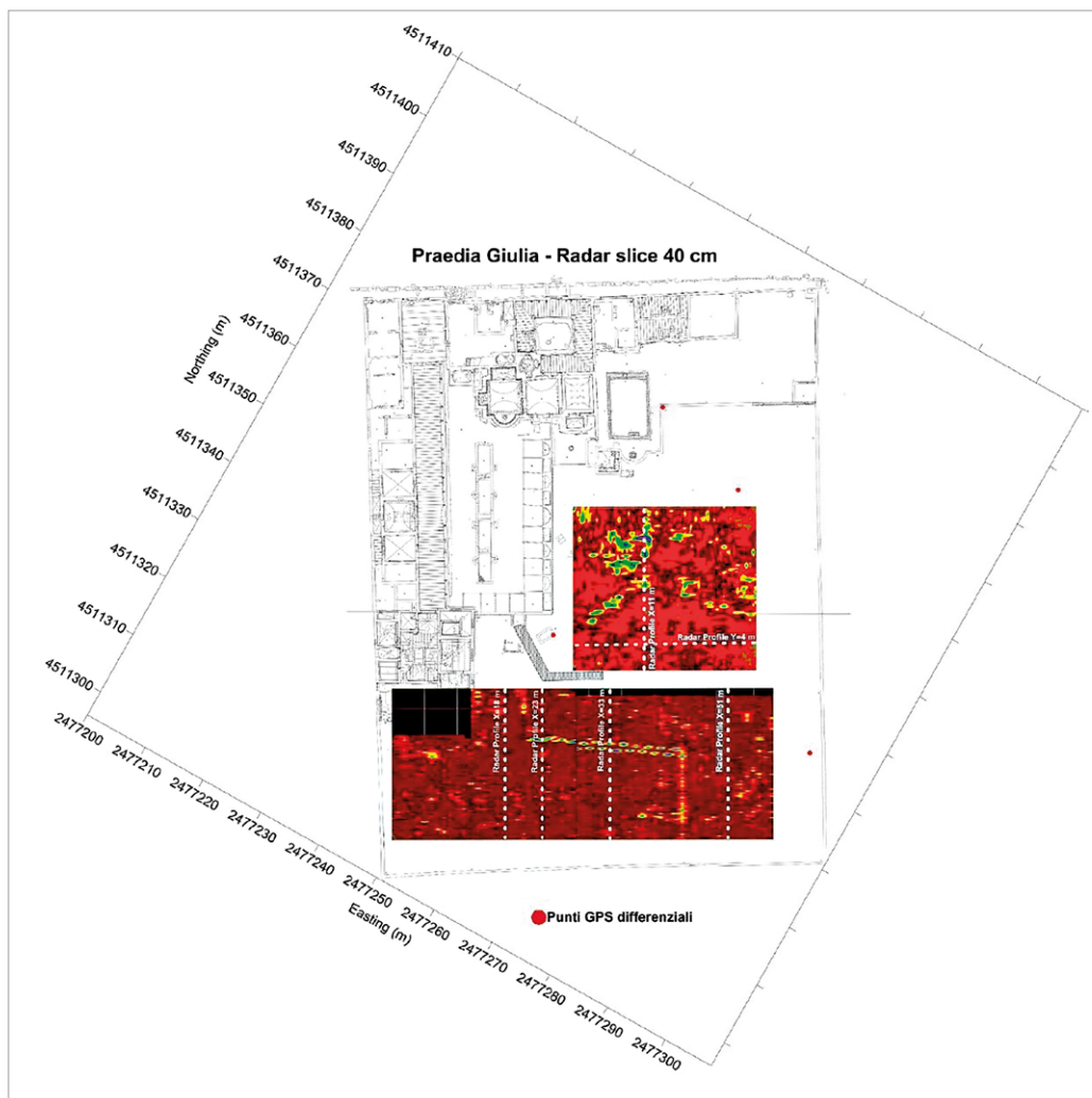
fig. 3. Mappa Praedia Iuliae Felicis: GPR-Slices Z=40 cm.
