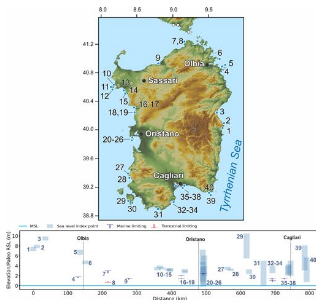
Figure 31. MIS 5 sea-level data for Sardinia (Italy). Upper panel: map of sites. The topography has been obtained from the SRTM void-filled DEM (Farr et al., 2007, NASA dataset). Lower panel: distance/elevation graph, counterclockwise around the island. Sites list: 1: Pedralonga (RSL ID 432); 2: Capo Monte Santu (RSL ID 435); 3: Orosei Nord (RSL ID 434); 4: Tavolara Punta la mandria (RSL ID 292); 5: Tavolara (RSL ID 431); 6: Capo Figari (RSL ID 430); 7: Capo Testa, Santa Reparata TLI (RSL ID 289); 8: Capo Testa, Santa Reparata MLI (RSL ID 290); 9: Badesi Mare San Pietro a Mare (RSL ID 300); 10: Cala Viola (RSL ID 388); 11: Capo Caccia 1 (RSL ID 382); 12: Capo Caccia 2 (RSL ID 383); 13: El tró (RSL ID 234); 14: Punta Padre Bellu (RSL ID 235); 15: Baurantinu (RSL ID 236); 16: Bosa Sect.1 (RSL ID 241); 17: Bosa Sect 2 (RSL ID 243); 18: Bosa Sect 3 (RSL ID 244); 19: Porto Alabe (RSL ID 238); 20: San Giovanni del Sinis (RSL ID 262); 21: San Giovanni del Sinis (RSL ID 271); 22: San Giovanni del Sinis (RSL ID 272); 23: San Giovanni del Sinis (RSL ID 265); 24: Faro Capo San Marco (RSL ID 266); 25: Capo San Marco (RSL ID 261); 26: San Giovanni del Sinis (RSL ID 263); 27: Buggerru (RSL ID 437); 28: Masua (RSL ID 436); 29: Sant'Antioco Cala Sapone (RSL ID 296); 30: Sant'Antioco (RSL ID 433); 31: Capo Malfatano (RSL ID 295); 32: Nora (RSL ID 1336); 33: Nora Is Fradis (RSL ID 1337); 34: Nora-Is Fradis (RSL ID 279); 35: Sa Illetta (RSL ID 278); 36: Cagliari Marina Piccola (RSL ID 1338); 37: Cagliari Cala Mosca (RSL ID 132); 38: Is Arenas (RSL ID 276); 39: Capo Carbonara Villasimius (RSL ID 293); 40: Capo Carbonara Isola dei cavoli-Cala Ponente (RSL ID 294).
