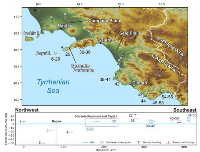
Figure 20. MIS 5 sea-level data for Campania (Italy). Upper panel: map of sites. The topography has been obtained from the SRTM void-filled DEM (Farr et al., 2007, NASA dataset). Lower panel: distance/elevation graph, from northwest (left) to southeast (right). Sites list: 1: Cellole Aurunci Masseria Transitiello (RSL ID 3624); 2: San Marcellino well (RSL ID 722); 3: San Marco Evangelista (RSL ID 739); 4: Sarno well (RSL ID 790); 5: Mitigliano (RSL ID 3581); 6: Scoglio Ricotta (I) Capri (RSL ID 821); 7: Scoglio Ricotta (II) Capri (RSL ID 822); 8: Grotta Testa del Cavallo Capri (RSL ID 800); 9: Grotta Jannarella Capri (RSL ID 801); 10: P.ta Campitiello Capri (RSL ID 802); 11: Cala del Limmo Capri (RSL ID 803); 12: Cala Articola (II) Capri (RSL ID 805); 13: Cala Articola (I) Capri (RSL ID 804); 14: Cala Articola (III) Capri (RSL ID 806); 15: Grotta Verde (I) Capri (RSL ID 807); 16: Grotta Verde (II) Capri (RSL ID 808); 17: Gr. Belvedere Capri (RSL ID 809); 18: Gr. Fontolina Capri (RSL ID 810); 19: I Faraglioni Capri (RSL ID 811); 20: Porto di Tragara (I) Capri (RSL ID 812); 21: Porto di Tragara (II) Capri (RSL ID 813); 22: P.ta di Masullo Capri (RSL ID 814); 23: a vascio funno Capri (RSL ID 815); 24: Cala Matermiana Capri (RSL ID 816); 25: Gr. Bianca (I) Capri (RSL ID 817); 26: Gr. Bianca (II) Capri (RSL ID 818); 27: P.ta della Chiavica Capri (RSL ID 819); 28: P.ta del Monaco Capri (RSL ID 820); 29: Cala di Ieranto (RSL ID 721); 30: Vettica Maggiore (RSL ID 823); 31: Grotta dello Smeraldo (RSL ID 798); 32: Conca dei Marini (III) Site I (RSL ID 767); 33: Conca dei Marini (II) Site I (RSL ID 766); 34: Conca dei Marini (I) Site I (RSL ID 720); 35: Conca dei Marini (V) (RSL ID 3623); 36: Conca dei Marini (IV) Site I (RSL ID 3565); 37: Ponte Barizzo (RSL ID 769); 38: Gromola (RSL ID 770); 39: Licosa Cape (III) (RSL ID 728); 40: Licosa Cape (II) (RSL ID 727); 41: Licosa Cape (I) (RSL ID 726); 42: Ogliastro Marina Baia Arena (RSL ID 592); 43: Palinuro Lido Ficocella (RSL ID 593); 44: Palinuro Cape (RSL ID 732); 45: The Riparo Infreschi cave (I) (RSL ID 3568); 46: The Riparo Infreschi cave (II) (RSL ID 3569); 47: The Riparo Infreschi cave (III) (RSL ID 3570); 48: The Riparo Infreschi cave (VI) (RSL ID 3573); 49: The Riparo Infreschi cave (IX) (RSL ID 3576); 50: The Riparo Infreschi cave (VIII) (RSL ID 3575); 51: The Riparo Infreschi cave (VII) (RSL ID 3574); 52: The Riparo Infreschi cave (V) (RSL ID 3572); 53: The Riparo Infreschi cave (IV) (RSL ID 3571); 54: Sapri (II) (RSL ID 792); 55: Sapri (RSL ID 791).
